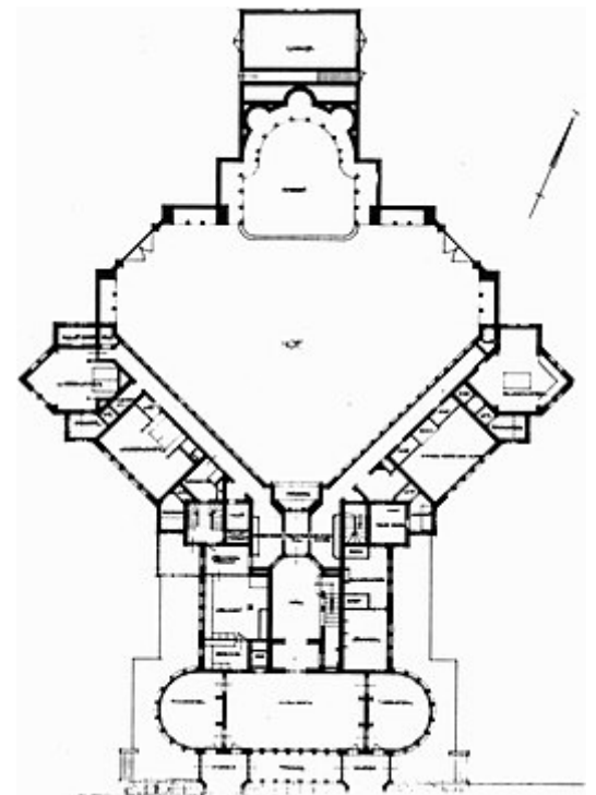
H.P. Berlage, eerste ontwerp
